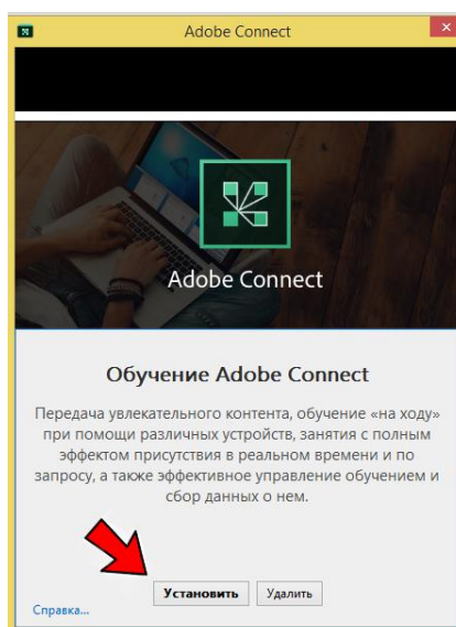
Рисунок 9 – Установка программы
